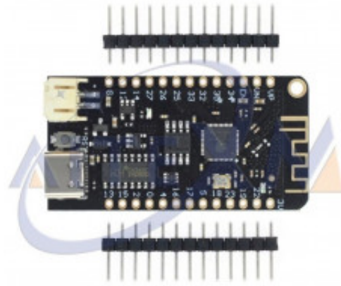
ESP32 REV1 - TYPE-C USB
